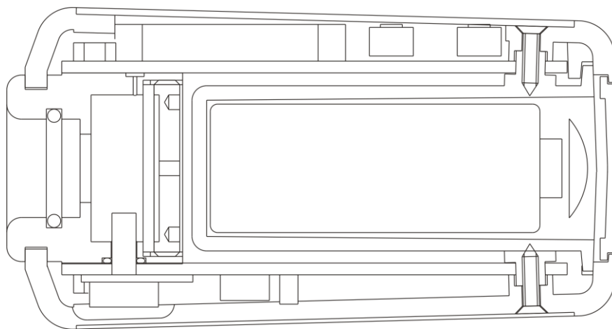
Fig. 3 Costruzione meccanica del calibratore (sezione).
