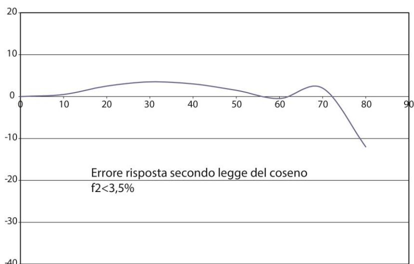
Fig. 3.2: errore direzionale
