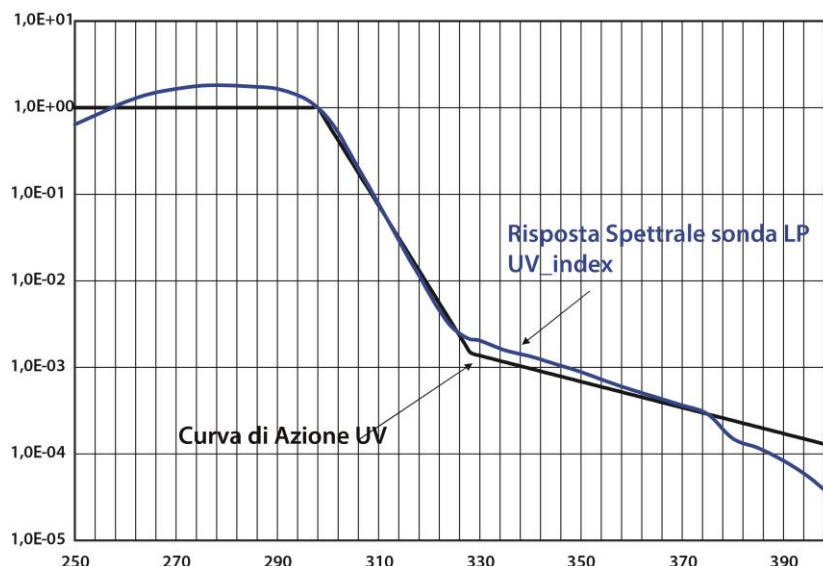
Fig. 3.1: risposta spettrale
