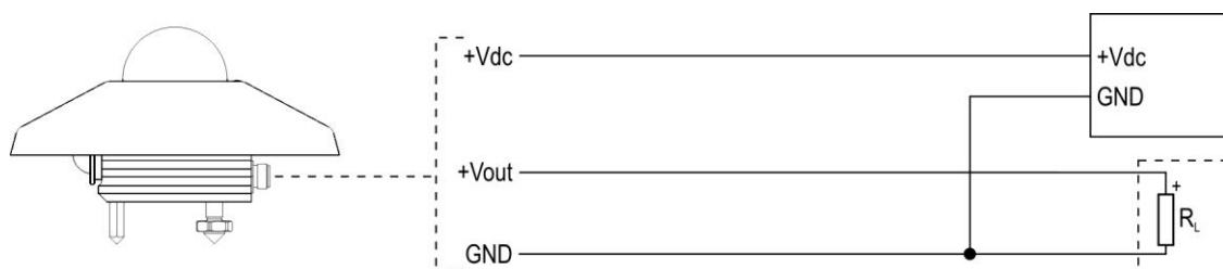
Fig. 4.4: connessioni LPUVI02...AV...
