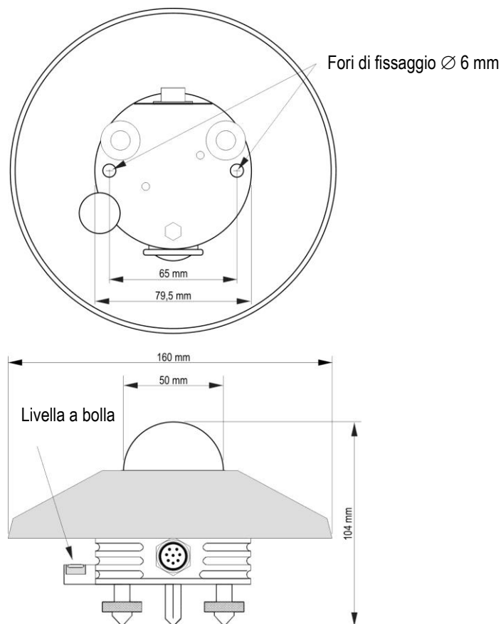
Fig. 4.2: fori di fissaggio e livella a bolla
