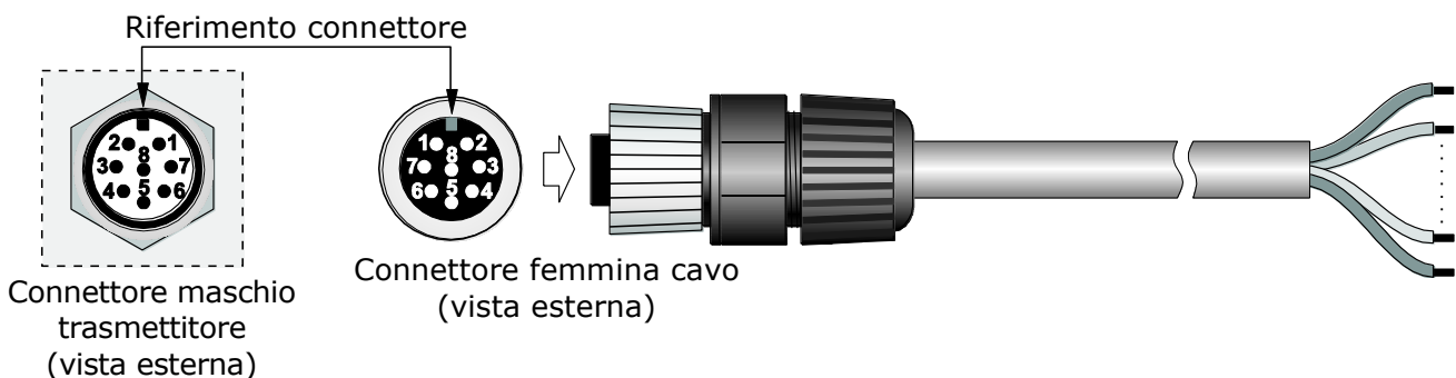
Fig. 3.2: piedinatura connettori
