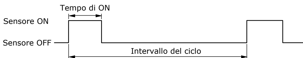
Fig. 4.1: Modalità di misura a intervalli ciclici
